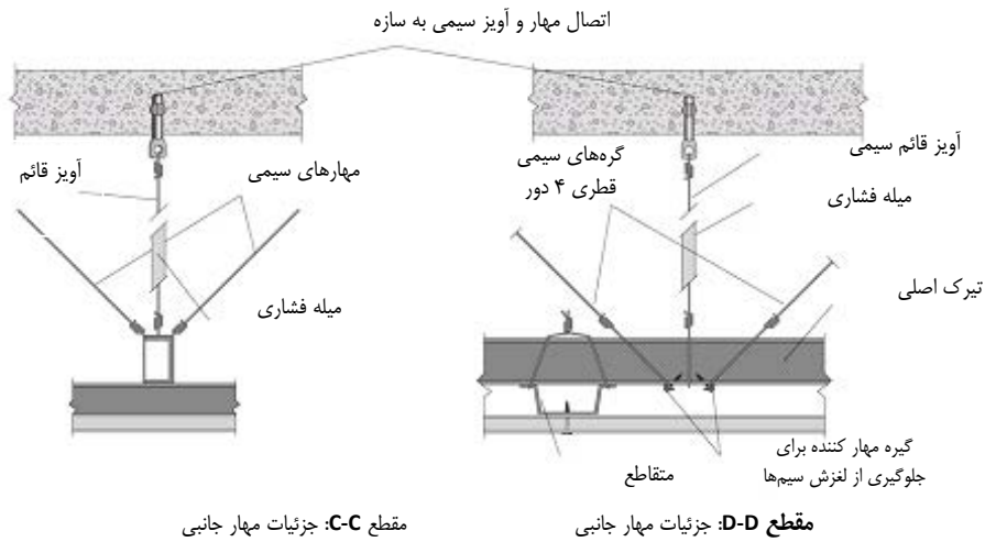
شکل پ-۳۴-۶- جزئیات مهاربندی جانبی برای سقف پانل گچی معلق مقاطع نشان داده شده در شکل پ-۶-۲۸
